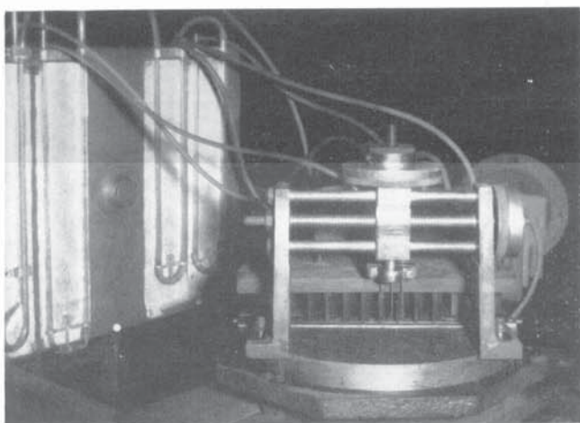
BLADE CASCADE TEST RIG
