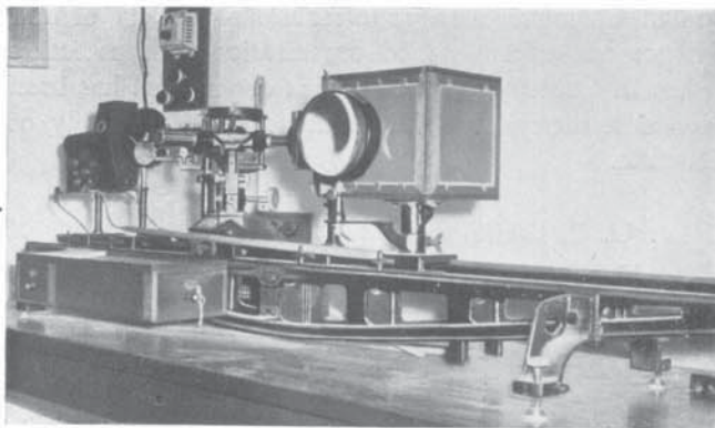
REICHART METALLOGRAPH
